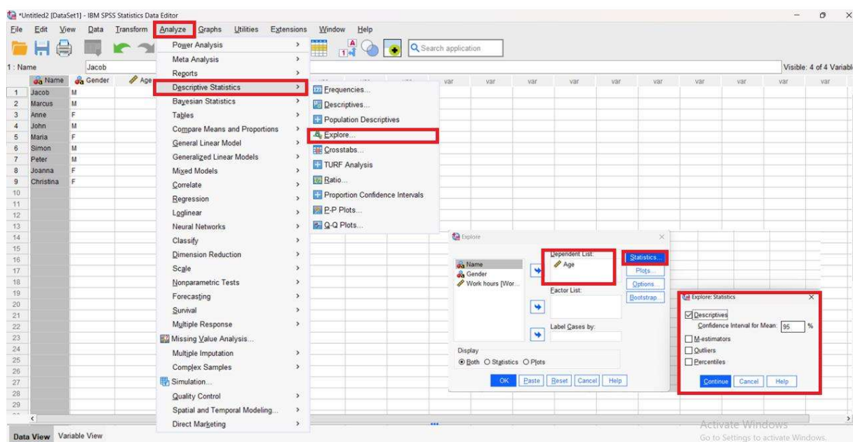
Rysunek 7.3 Ustawienia statystyk opisowych
