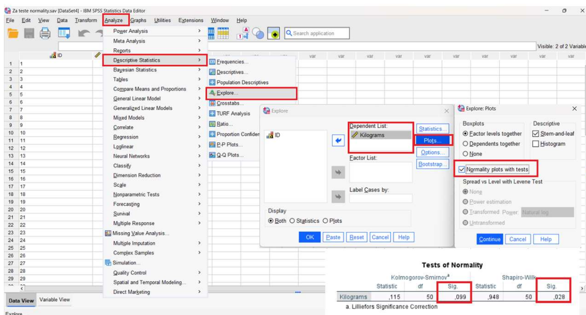
Rysunek 7.11 Ustawienia i wyniki testu normalności
