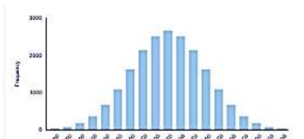
Slika 2.1 Primer Gaussove distribucije ili zvonaste krive
