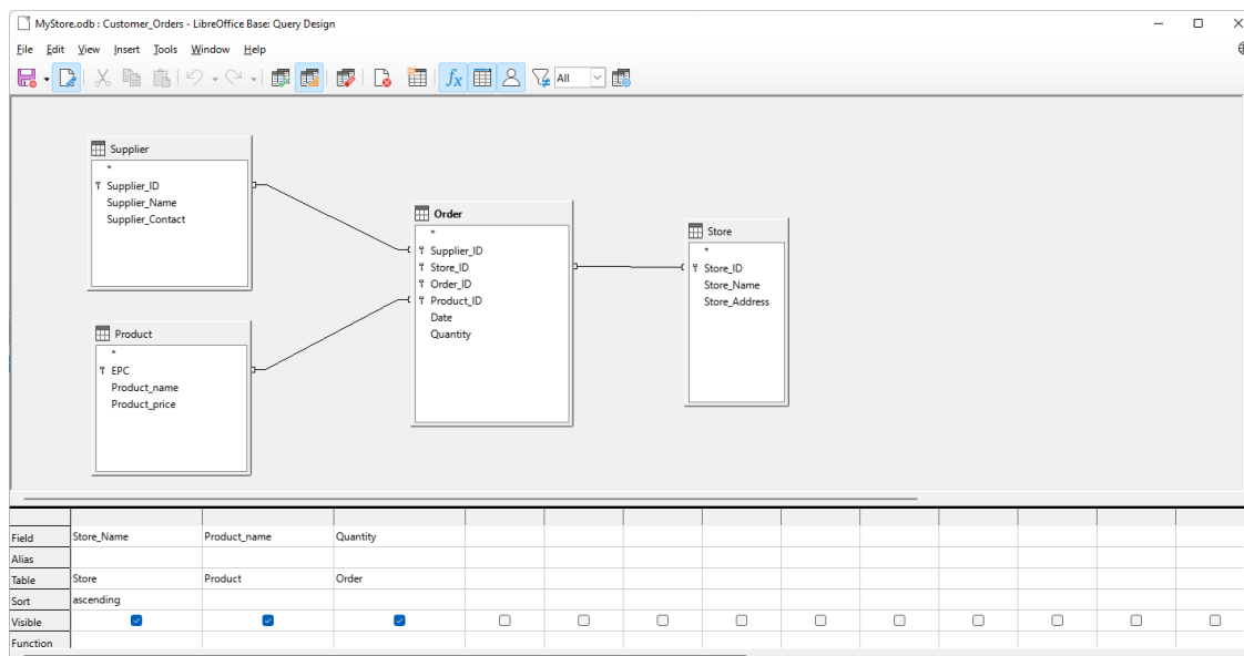
Slika 3.4 QBE upit ekvivalentan gornjem SQL upitu.
