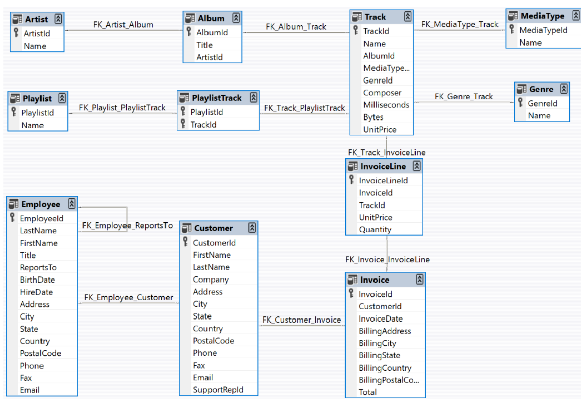
Slika 8.4 Model podataka baze podataka Chinook.
