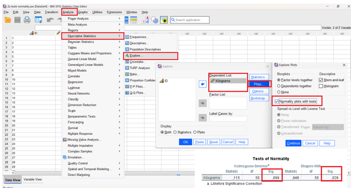
Slika 7.11 Postavke i rezultati testa normalnosti.
