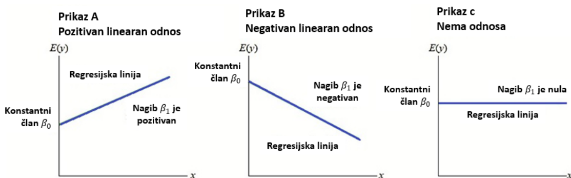
Slika 5.1 Primeri grafikona linearnog odnosa.
