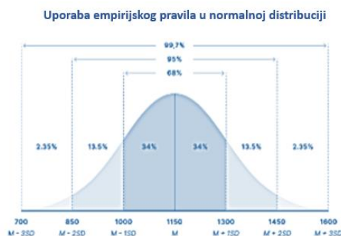
Slika 2.3 Empirijsko pravilo u normalnoj distribuciji.
