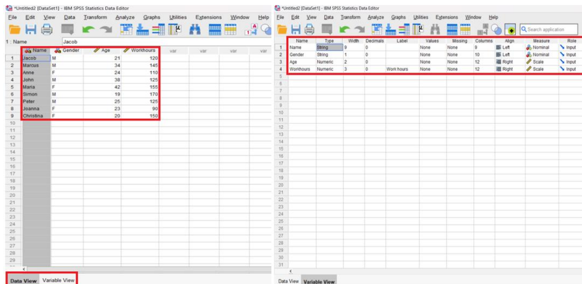
Slika 7.2 Prozori za prikaz podataka i varijabli.
