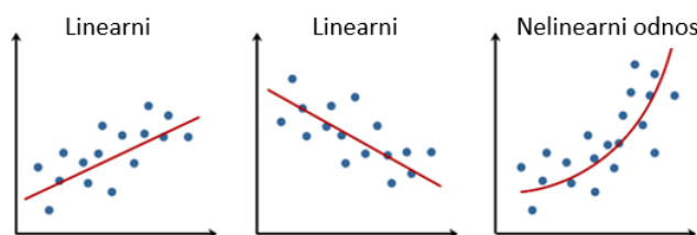
Slika 1.6 Grafikon jednostavne linearne regresije.
