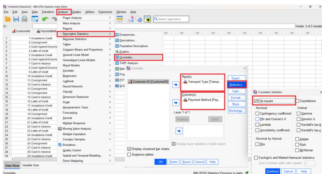
Slika 7.16 Postavke Hi-kvadrat testa.
