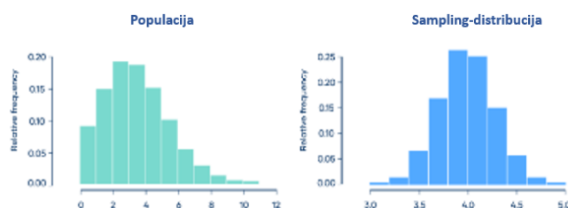
Slika 2.8 Primer populacije u Poissonovoj distribuciji i normalnoj distribuciji.
