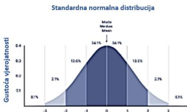
Slika 2.6 Grafikon standardne normalne distribucije.
