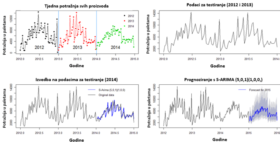
Slika 9.4 Obuka, testiranje i predviđena potražnja S-ARIMA (5,0,1)(1,0,0) 52 modela.
