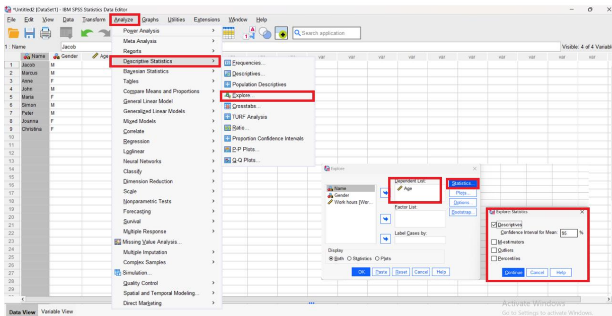
Slika 7.3 Postavke deskriptivne statistike.
