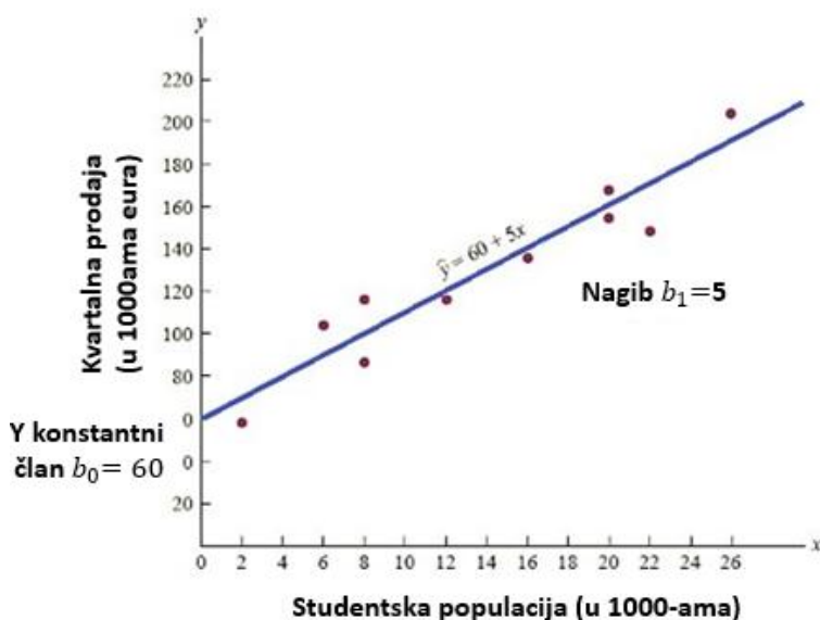
Slika 5.5 Dijagram rasipanja studentske populacije i tromesečne prodaje.
