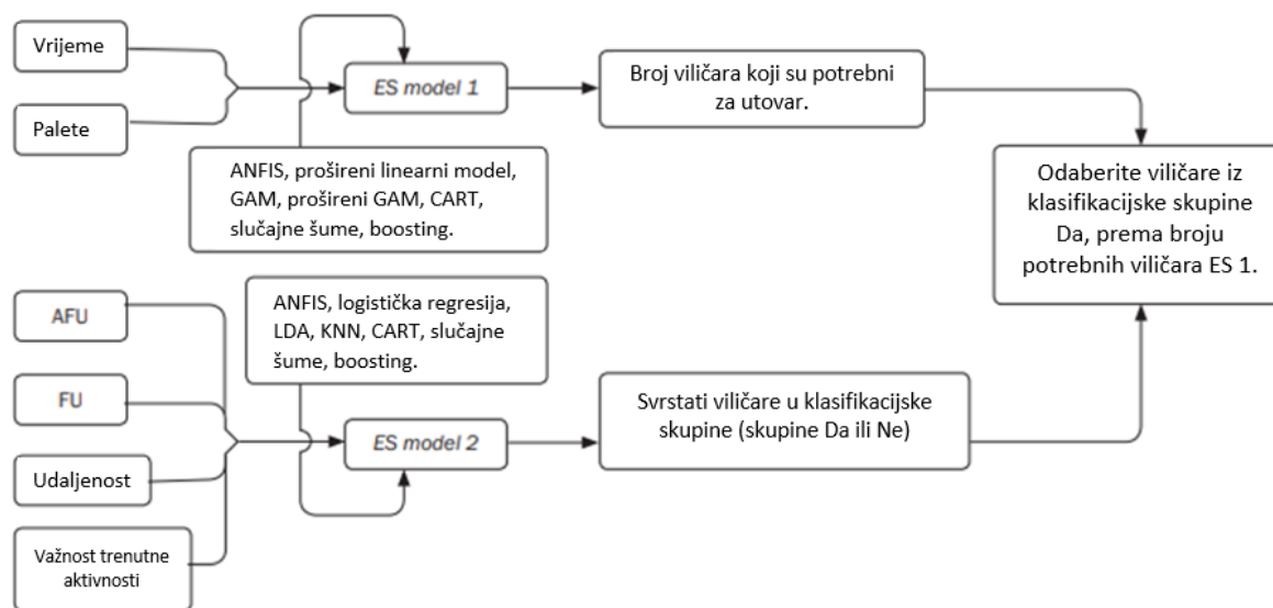
Slika 10.4 Izgradnja strukture skladišnog DSS-a na osnovu AI i ML algoritama.
