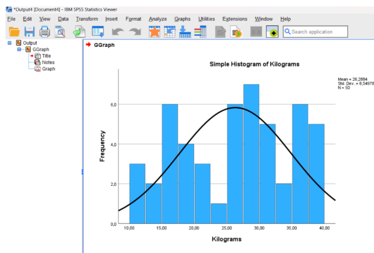
Slika 7.9 Histogram rezultata testa normalnosti.
