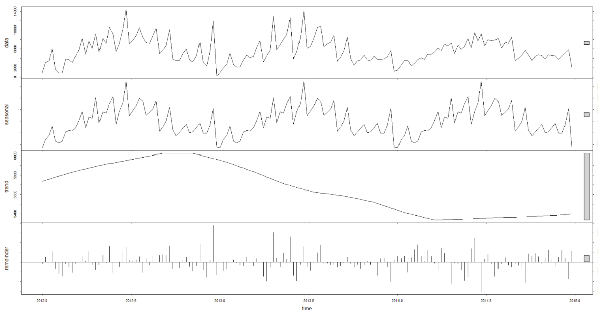
Slika 9.3 STL dekompozicija podataka o potražnji.
