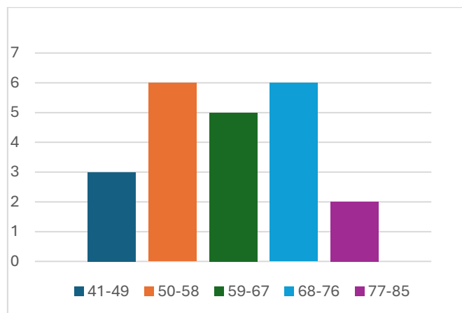
Slika 1.5 Grafikon distribucije frekvencija.
