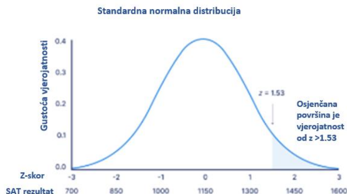
Slika 2.7 Standardna normalna distribucija s naznačenim SAT
