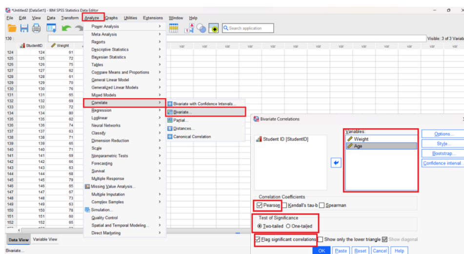
Slika 7.14 Postavke testa korelacije.
