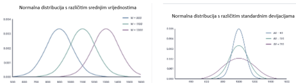
Slika 2.2 Normalna distribucija s različitim srednjim vrednostima i različitim standardnim devijacijama.
