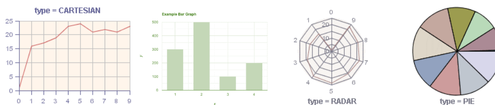
Slika 1.2 Primeri grafičkih prikaza podataka.
