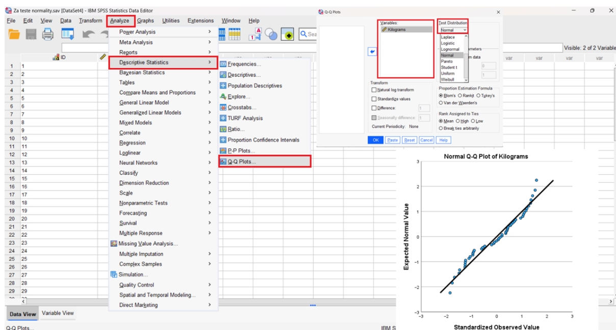
Slika 7.10 QQ grafikon test normalnosti - postavke i rezultati.
