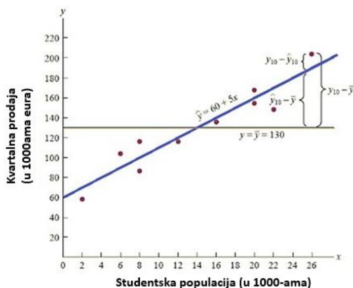
Slika 5.8 Regresiona linija u slučaju Best Burgera.
