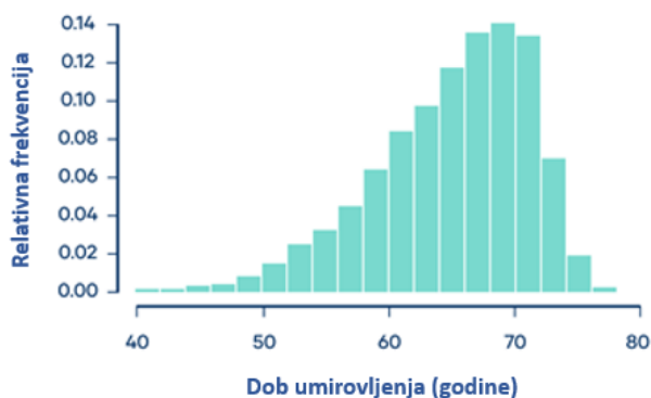
Slika 2.9 Grafikon kontinuirane distribucije.
