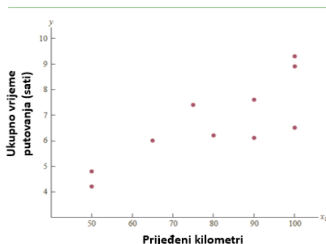
Slika 5.10 Dijagram rasipanja za Frigo transportnu kompaniju.
