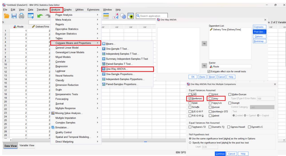
Slika 7.18 Postavke za ANOVA analizu.
