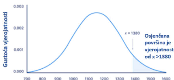
Slika 2.5 Grafikon funkcije gustine verovatnoće SAT rezultata.
